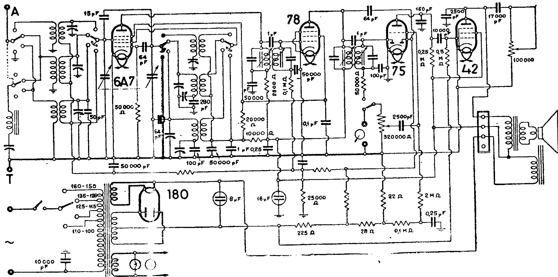
RADIOMARELLI - MOD. «ALCOR»
